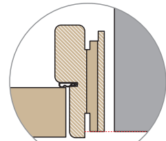
Установка коробки с прямыми наличниками
