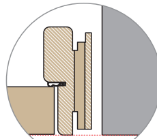
Установка коробки с телескопическими наличниками
