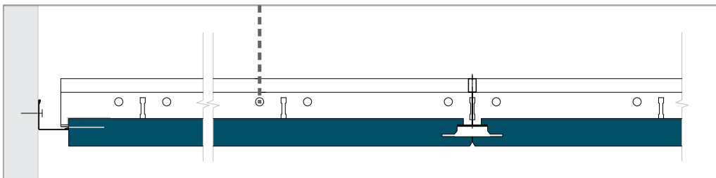
Отделка периметра с помощью пристенного уголка и кромочной клипсы для создания эффекта парящего края.
