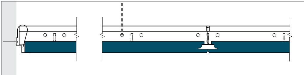
Отделка периметра с помощью алюминиевого теневого пристенного уголка и фиксирующей клипсы.
